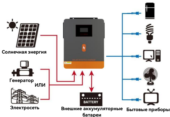
Рисунок 1. Гибридная система электроснабжения
