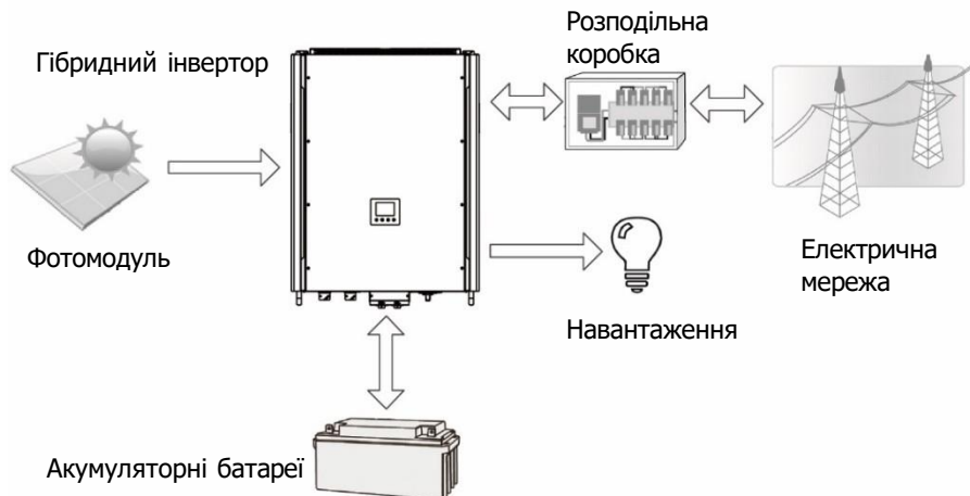
Малюнок 1 Базова схема роботи гібридного інвертора
