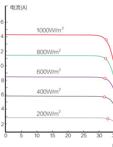
电流-电压曲线 (435W) Cells temp.=25°C
