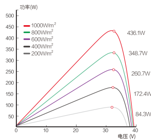
功率-电压曲线 (435W) Cells temp.=25°C
