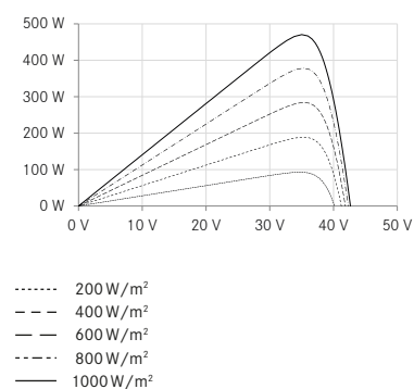
UP-diagram e.g. LX-470M/182-120+
